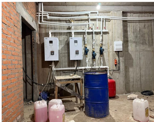
Узел временной системы отопления
