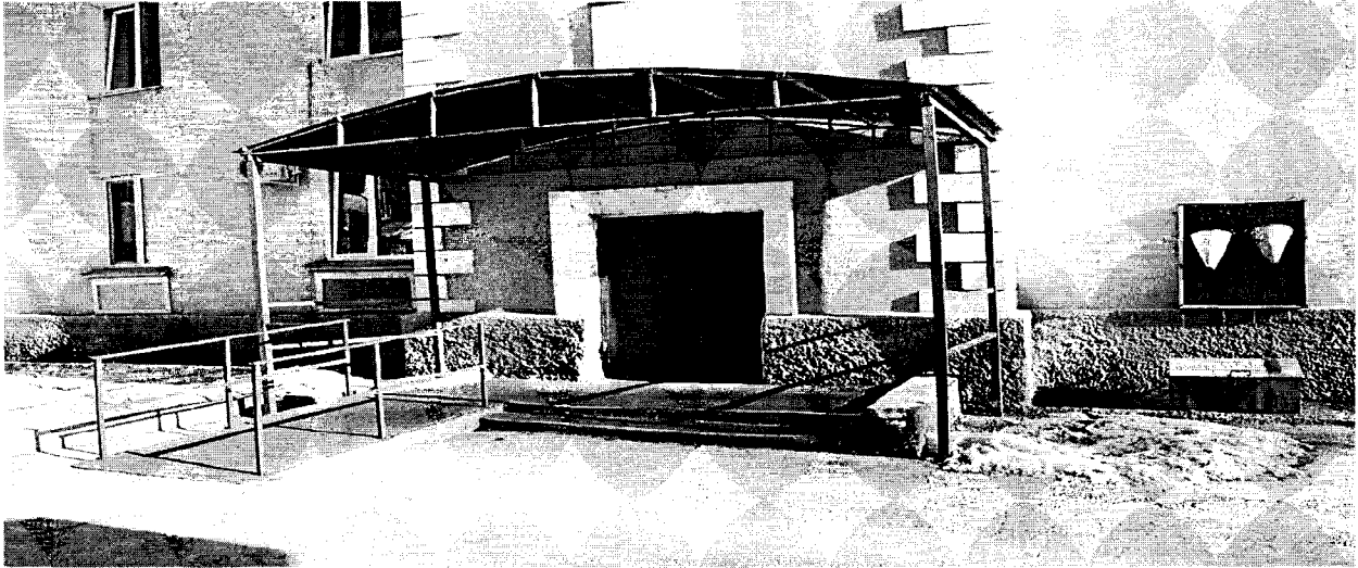
Оборудование пандуса в Партизанском психоневрологическом диспансере.
